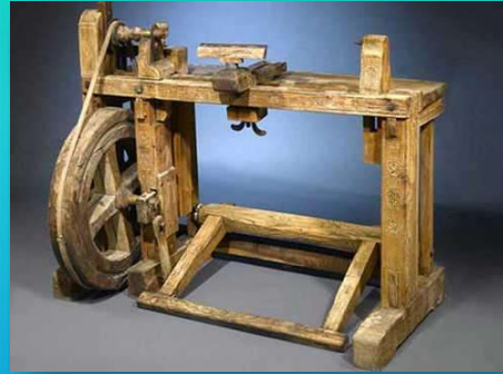
Старинный токарный станок с ножным приводом
